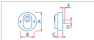
Schutzrosette MIT Zylinderabdeckung „Aussen“
