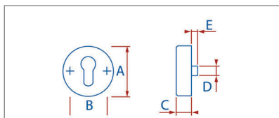
Schutzrosette OHNE Zylinderabdeckung „Aussen“
